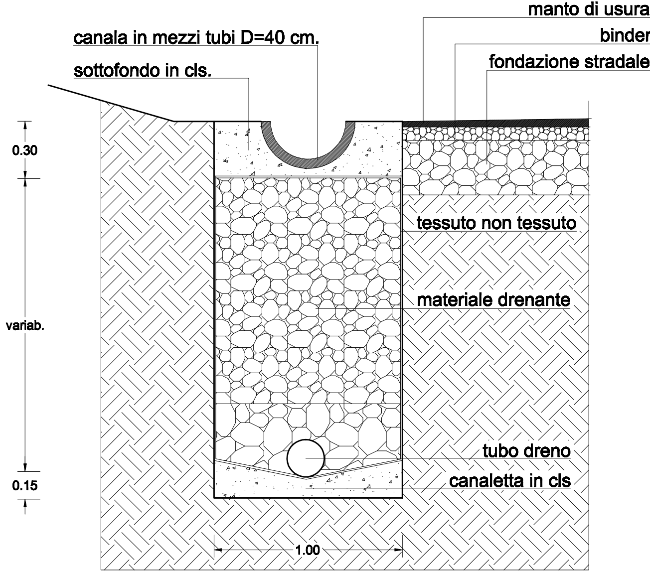
PARTICOLARE FOSSA DRENANTE E CANALA DI RACCOLTA ACQUE
